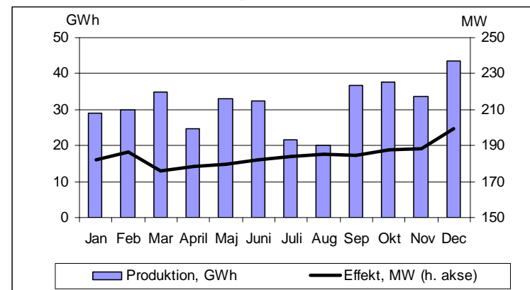
Figuren viser den månedlige produktion og installeret effekt i 2004.
